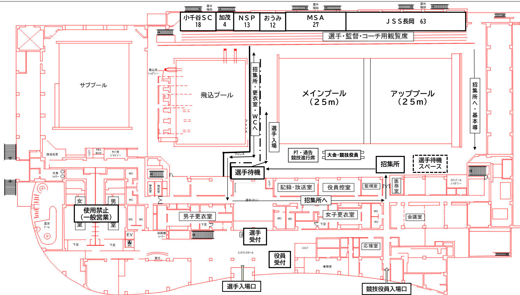
ダイエーフロビスフェニックスプール 1階平面図(長岡市親善記録)
