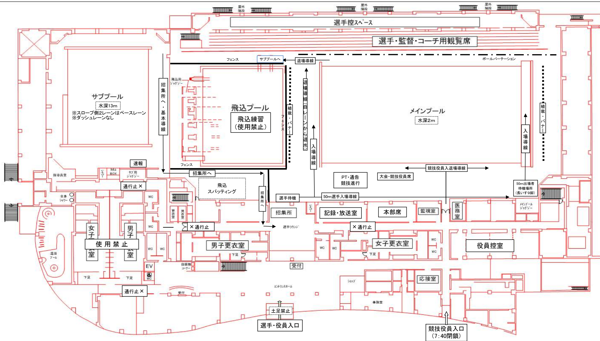
ダイエーフロビスフェニックスプール 1階平面図 (国体県予選会)
